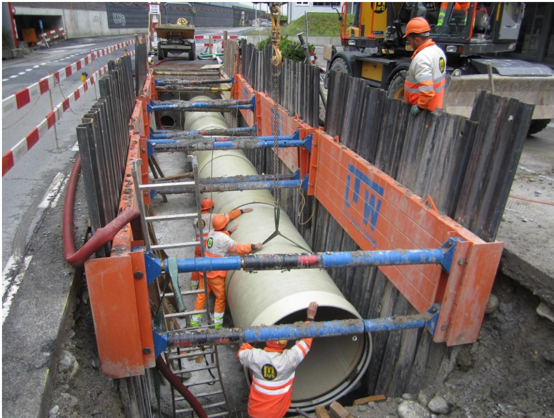
Bildlegende: Leitungsbau mittels Kammerplatten
